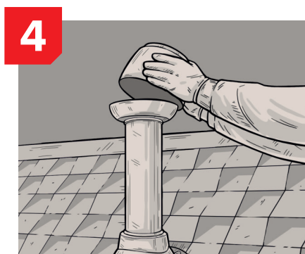
4 Установите защитный колпак. При установке вентиляционного выхода на канализационный стояк, необходимо удалить внутренний конус колпака.
