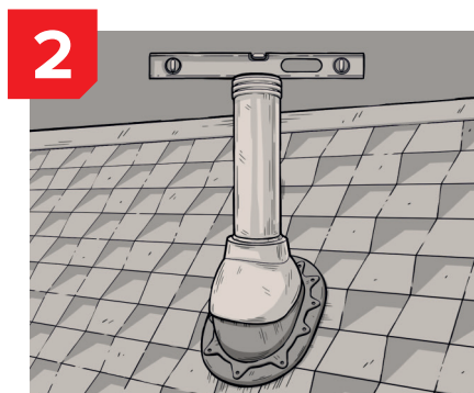
2 Установите вентиляционный выход на проходной элемент. Угол установки скорректируйте по строительному уровню.
