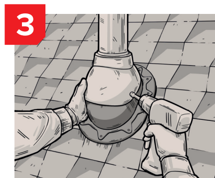
3 Зафиксируйте вентиляционный выход к проходному элементу кровельными саморезами. Рекомендуемое количество кровельных саморезов 6 штук.
